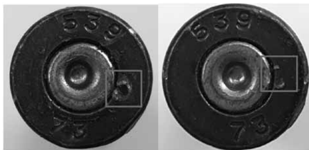
Рис. 3 Следы на донной части гильзы, стрелянной из карабина «РПД-О», от штифта, выполненного на патронном упоре затвора
